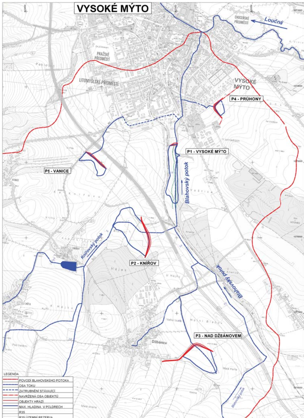
Protipovodňová opatření v okolí Blahovského potoka - červeně zakresleny suché poldry P1 až P5 (k článku na str. 15).
