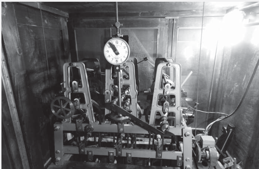
To jsou „střeva“ stroje na bývalém soudu.
