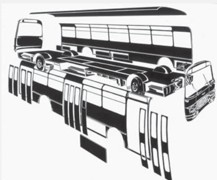
Panelová stavba autobusu Š 11.
