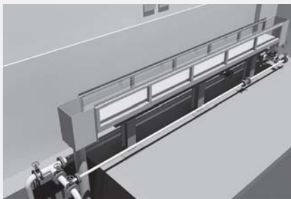
Vizualizace proskleného hydraulického měrného žlabu s přiváděcím potrubím.
